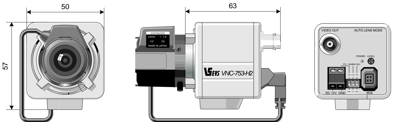
Рис.3. Камера VNC-753-H2
