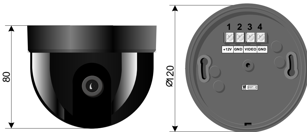
Рис.1. Камера VSS-731
